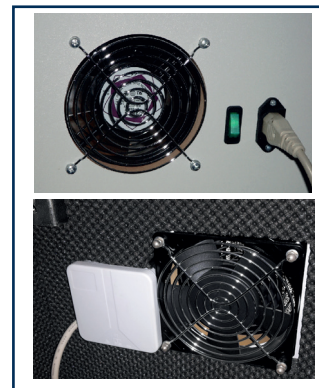
Kaltgeräteanschluß für Drucker und Ventilator
